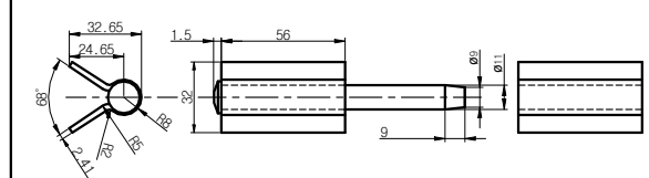
돌저귀 부품도
