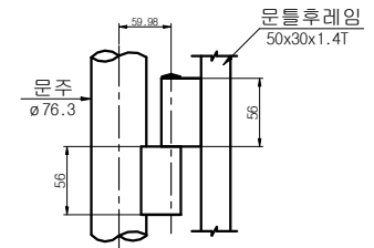
돌저귀 조립도
