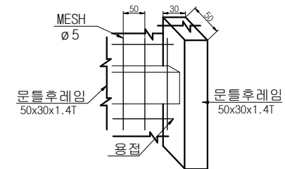
MESH 조립도
